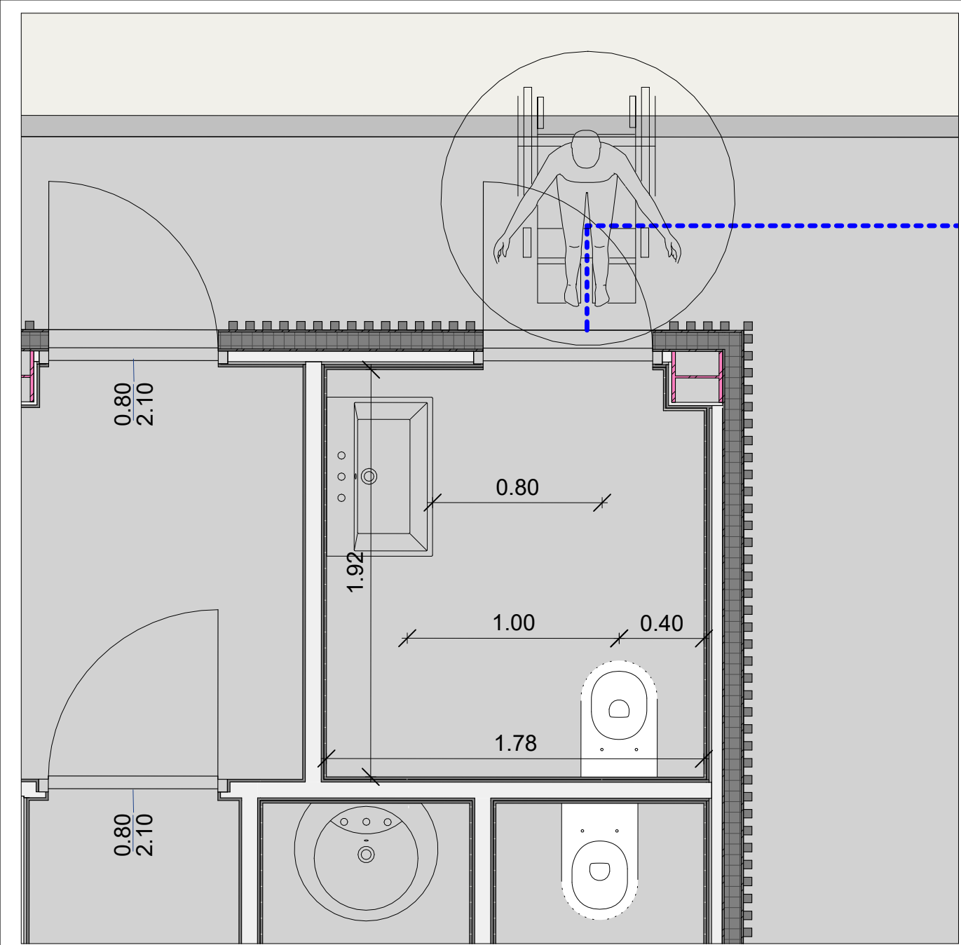
Percorsi legge 13/1989 Scala 1:25
