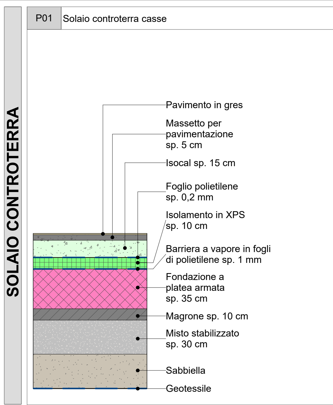
Abaco dei pacchetti Scala 1:20
