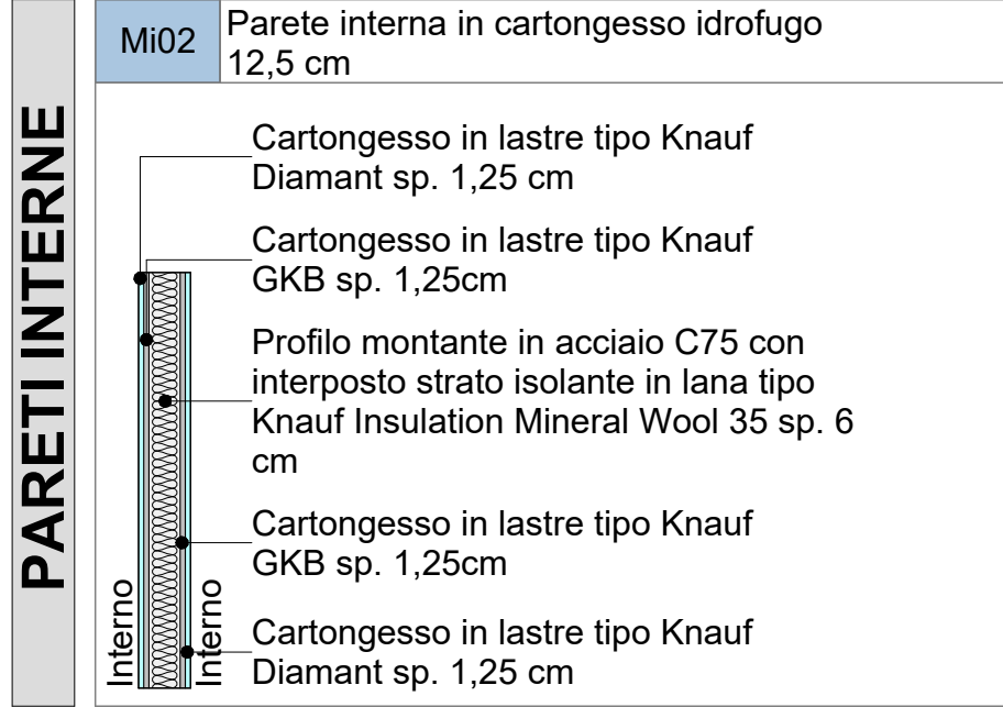
Abaco dei pacchetti Scala 1:20
