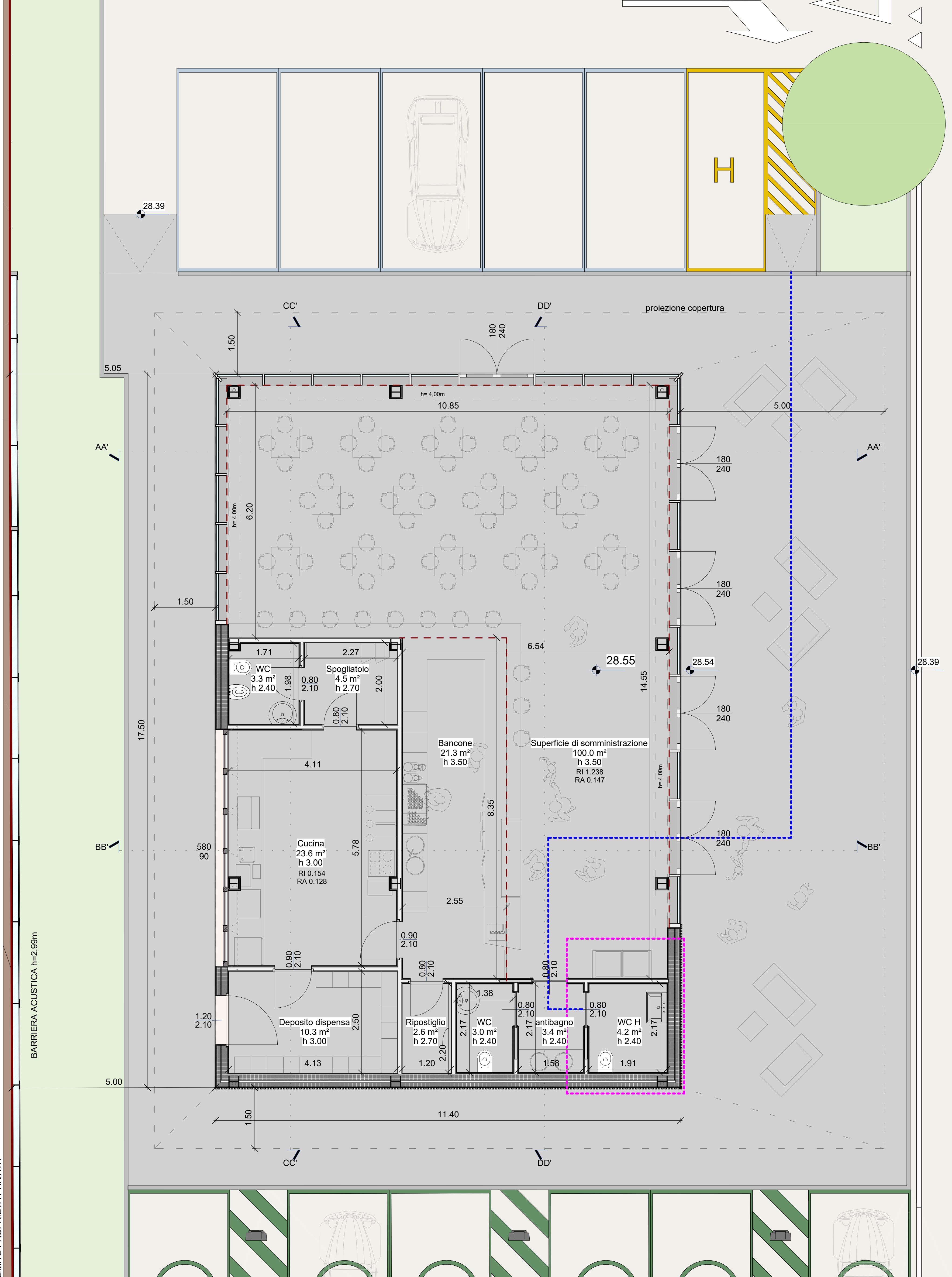
Piano terra Scala 1:50
