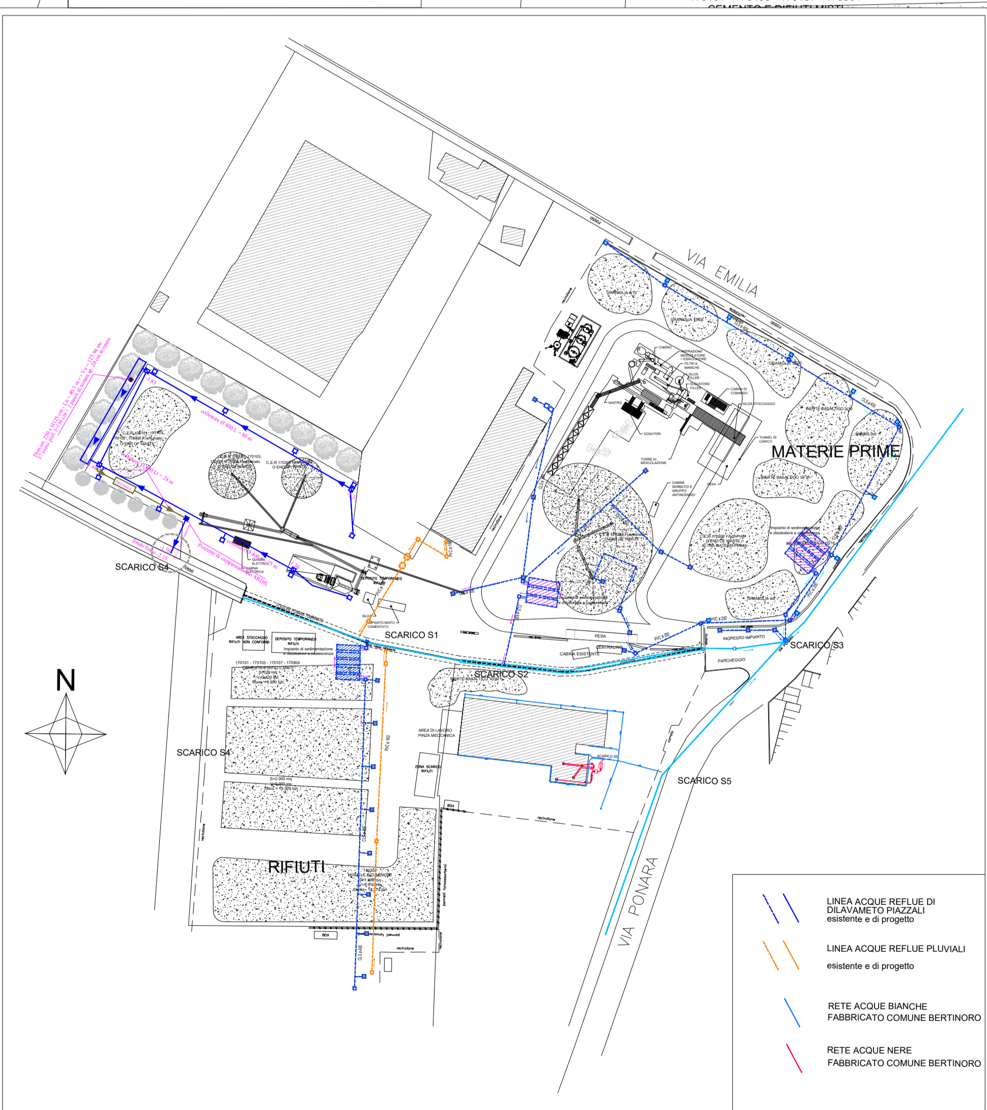
PLANIMETRIA FOGNATURE - STATO DI PROGETTO
