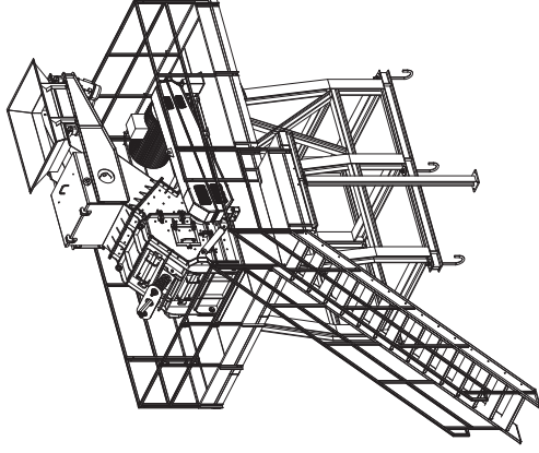
TELAIO SUPPORTO MULINO
