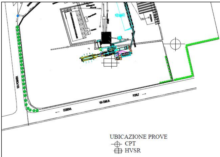
Fig. *. Ubicazione indagini Aprile 2018
