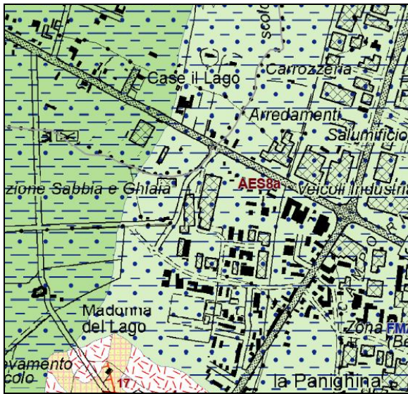
Fig. 3. Particolare Carta Geologica dell'Emilia Romagna
