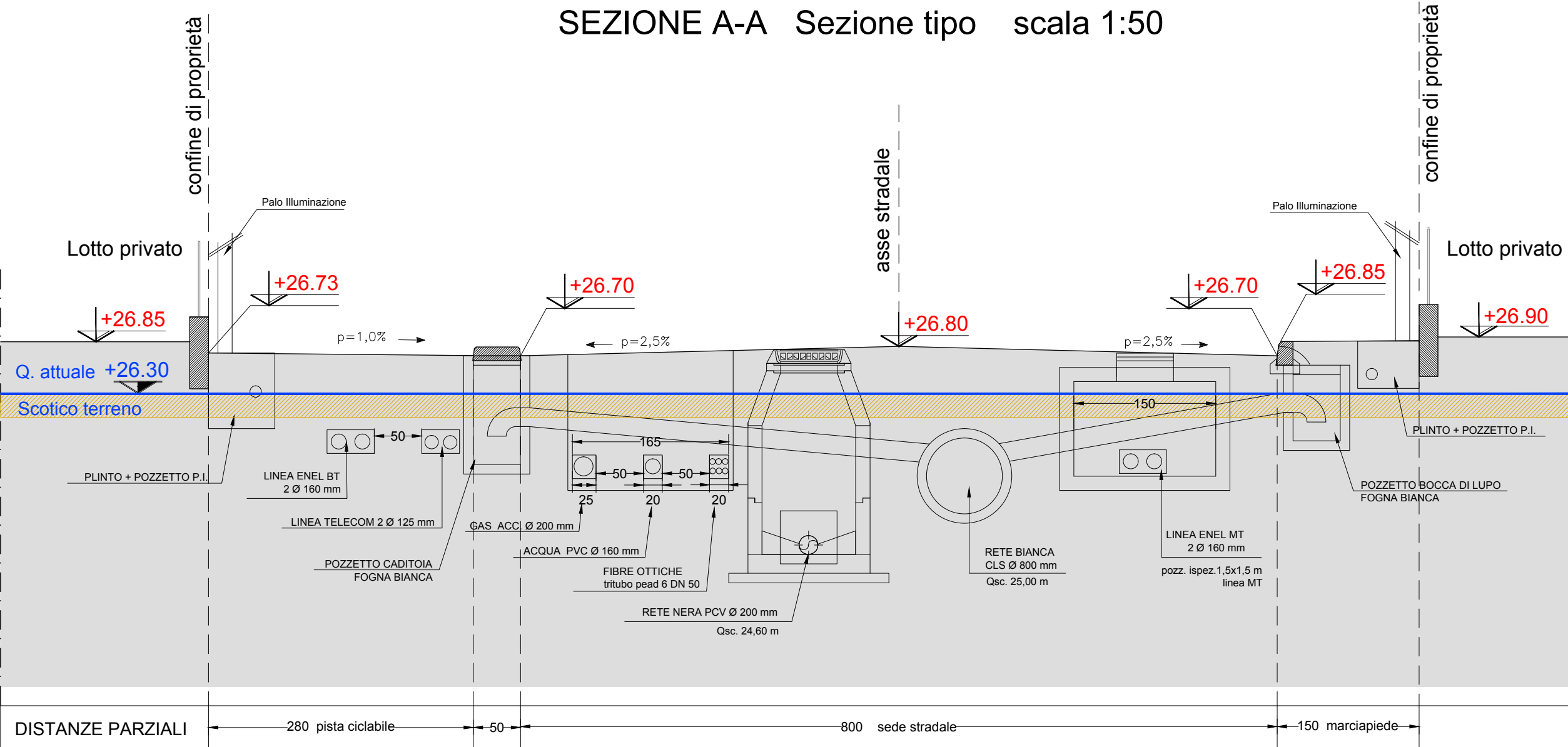
SEZIONE A-A Sezione tipo scala 1:50
