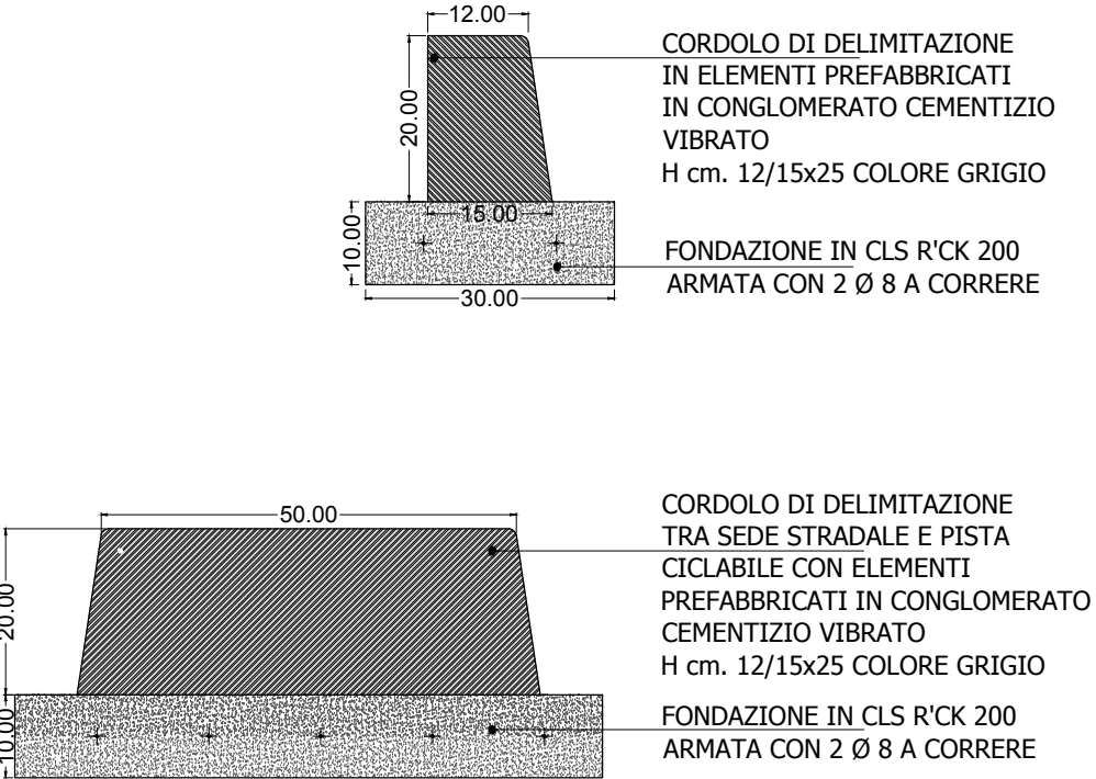
PARTICOLARE CORDOLI scala 1:10
