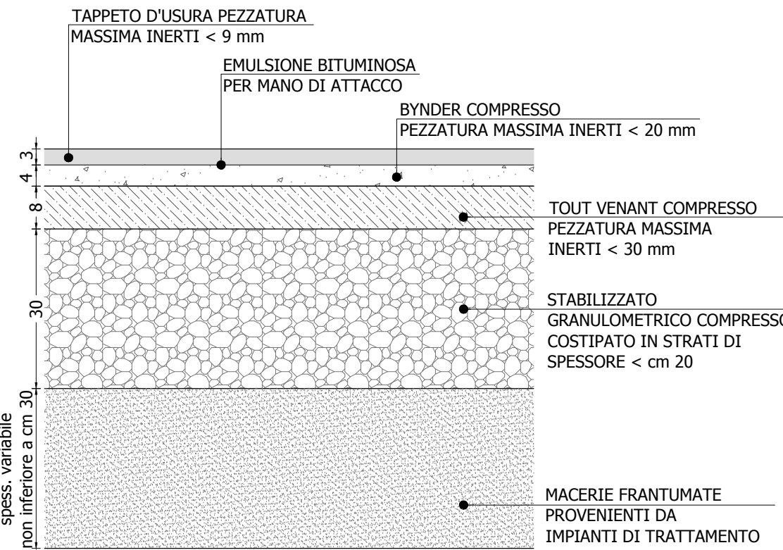
PACCHETTO STRADALE Spessore 75 cm circa scala 1:10
