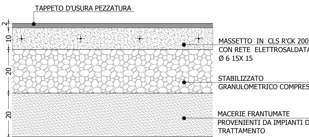
PACCHETTO MARCIAPIEDE Spessore 52 cm scala 1:10
