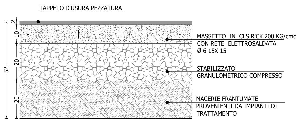
PACCHETTO MARCIAPIEDE Spessore 52 cm scala 1:10
