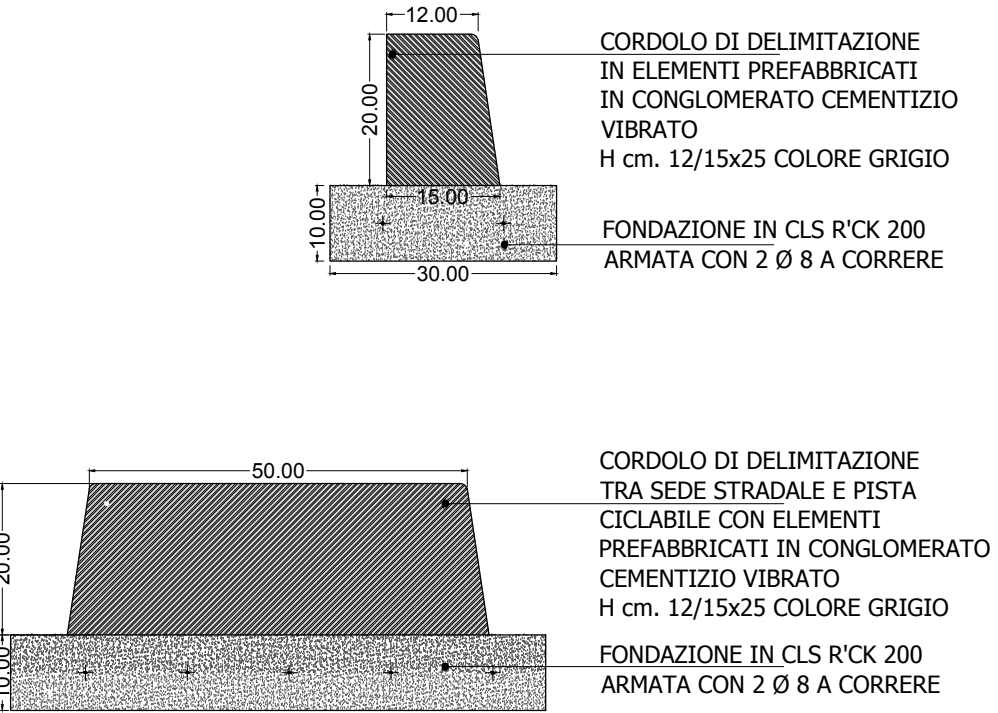
PARTICOLARE CORDOLI scala 1:10
